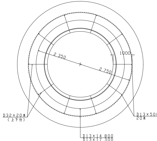
鉄筋組立図 S=1:100
