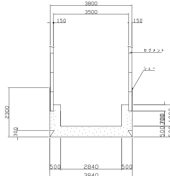
コンクリート集水井槽 S=1:100
