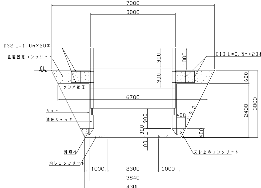
刃口金物（沓）据付工 S=1:100
