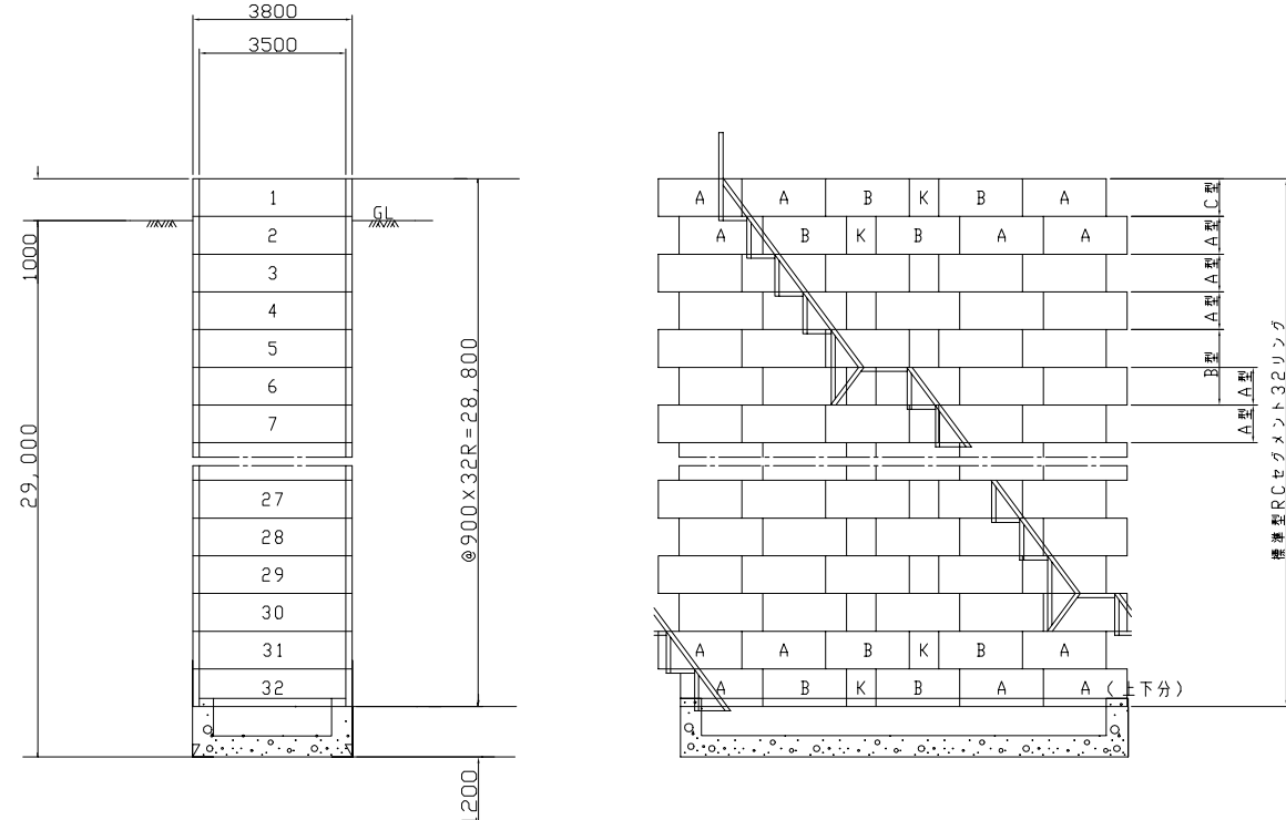
コンクリート集水井槽 S=1:100
